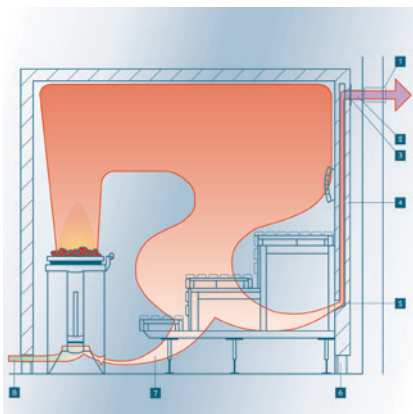
Abbildung: Ausreichender Luftaustausch mit Hilfe eines zugfreien Lüftungssystems. Quelle: CIRCO THERM von Klafs
