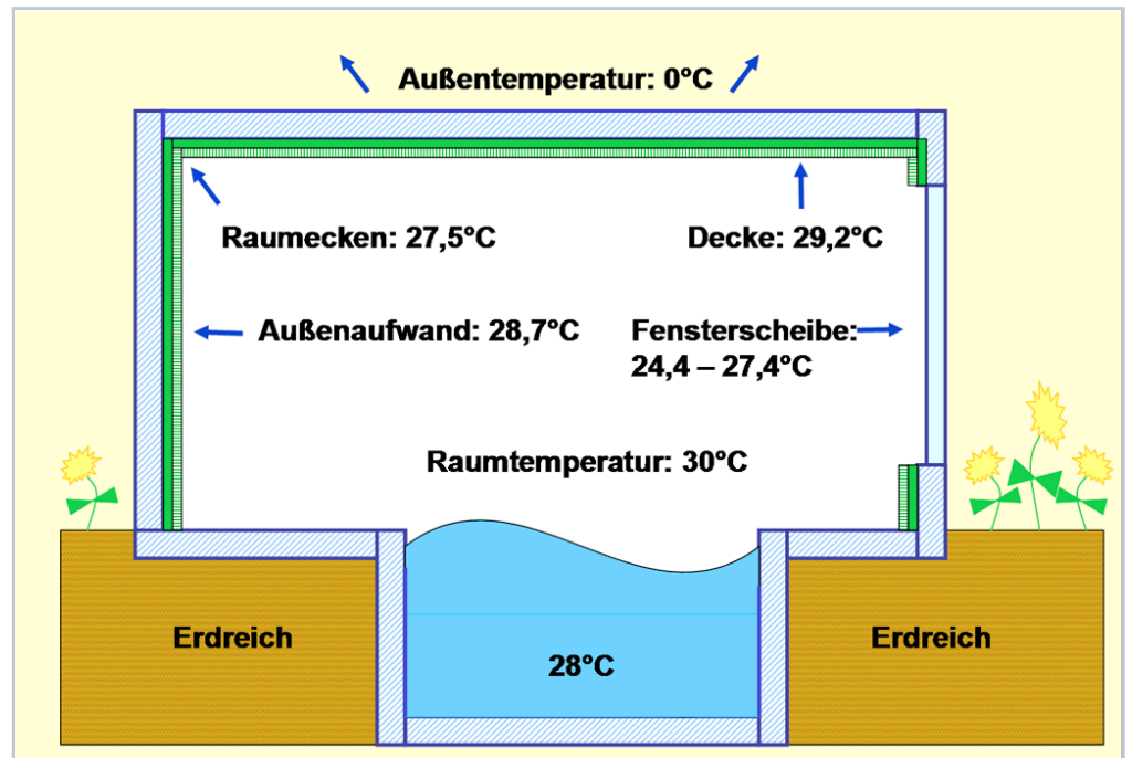
Abbildung: Oberflächen-Temperaturen in wärmedämmten Schwimmhallen Quelle: abgeändert nach EN-OP Institut
