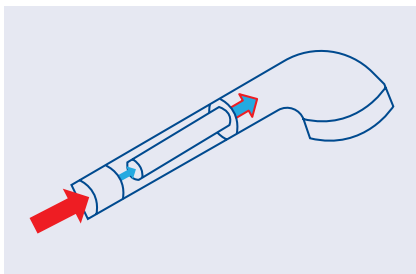
Abbildung: Brause, die Luft ansaugt und mit Wasser mischt (Preis: circa 8 Euro für den Sparduschkopf).
